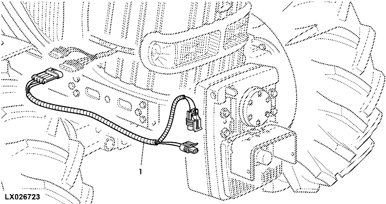
프론트 PTO 와이어링 하니스
