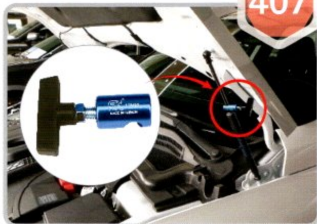
후드(쇼버) 고정기
