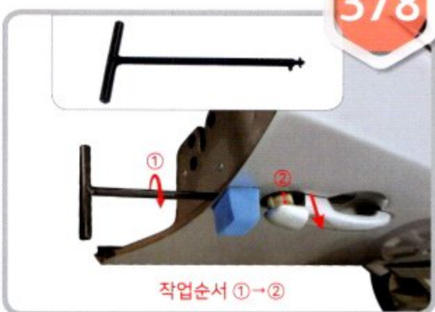
도어캐처 렌치
